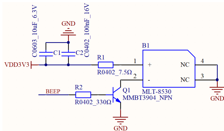
图 2-2 蜂鸣器电路示意
