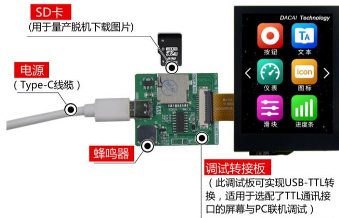
图 1-5 调试工具图
