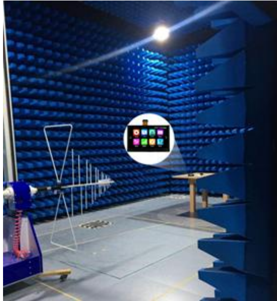
图 5-4 RE 测试图
