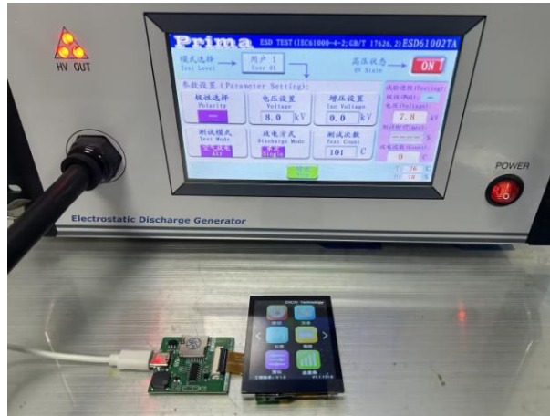
图 5-2 ESD 测试图
