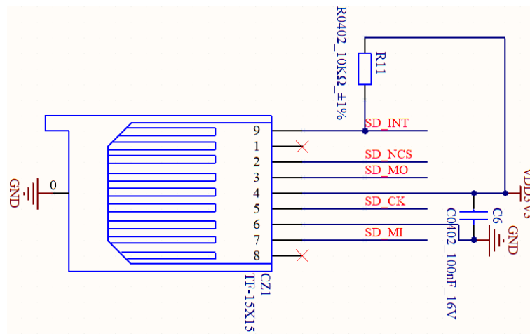
图 2-3 SD 卡座电路示意
